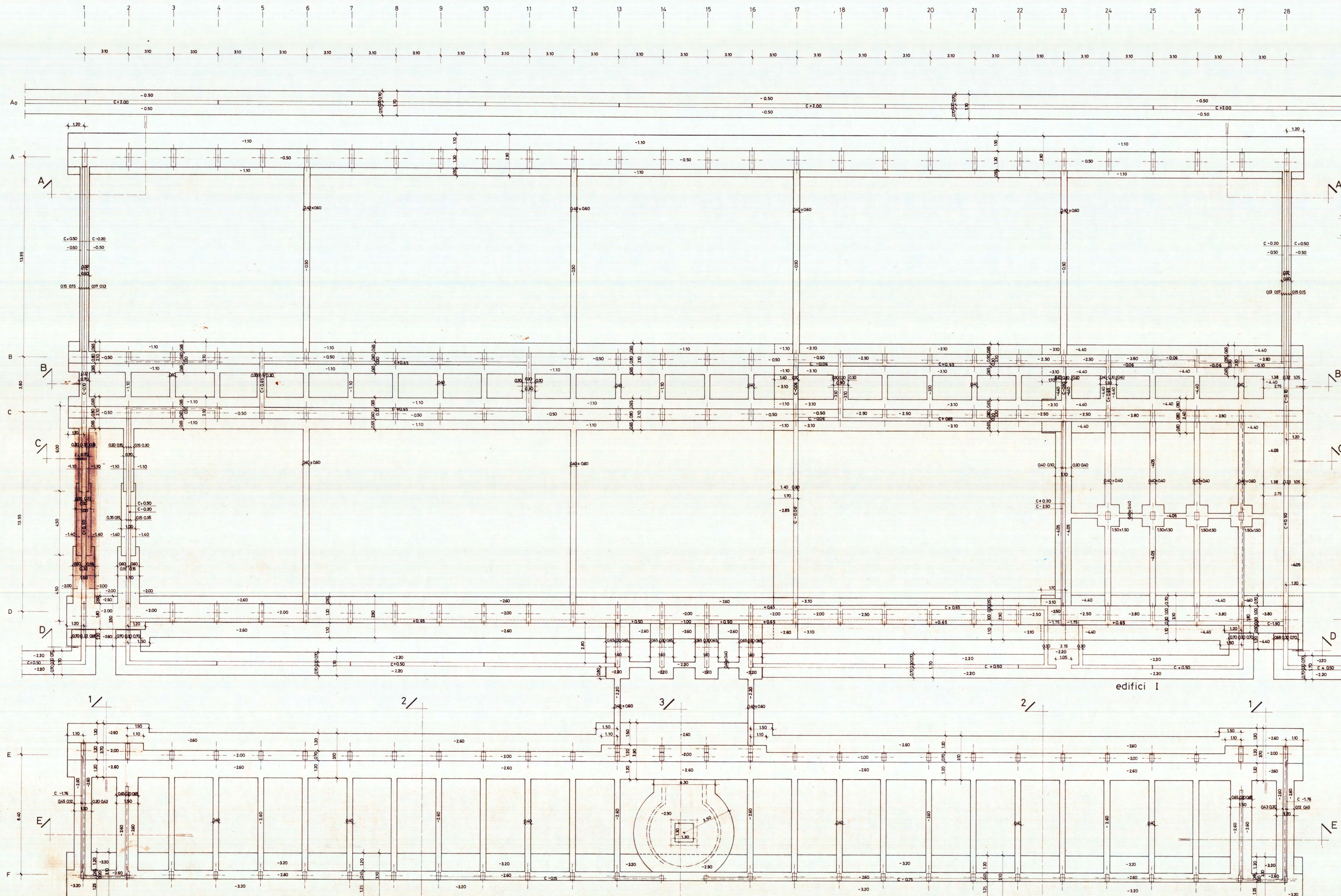
PLANTA FONAMENTS E: 1/100
