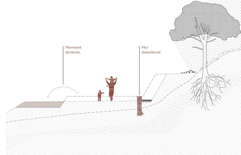
SECCIÓ - PROPOSTA
