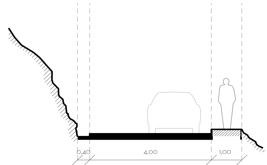
Secció BC
